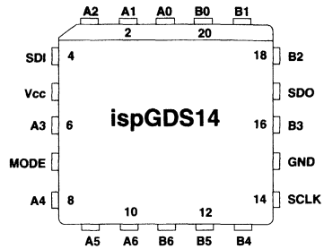
20-Pin PLCC
